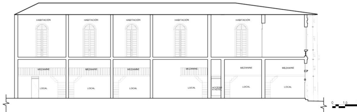
Corte longitudinal
